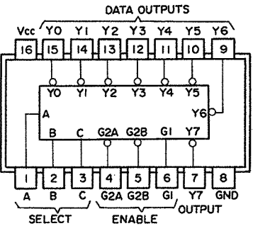
'LS138, FUNCTION TABLE
